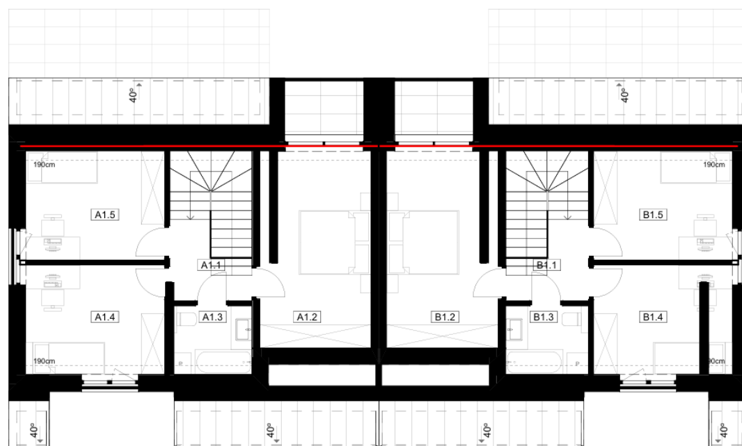
RZUT PODDASZA
