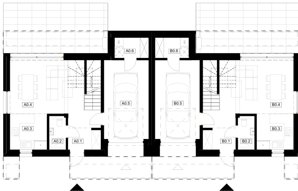
RZUT PARTERU
