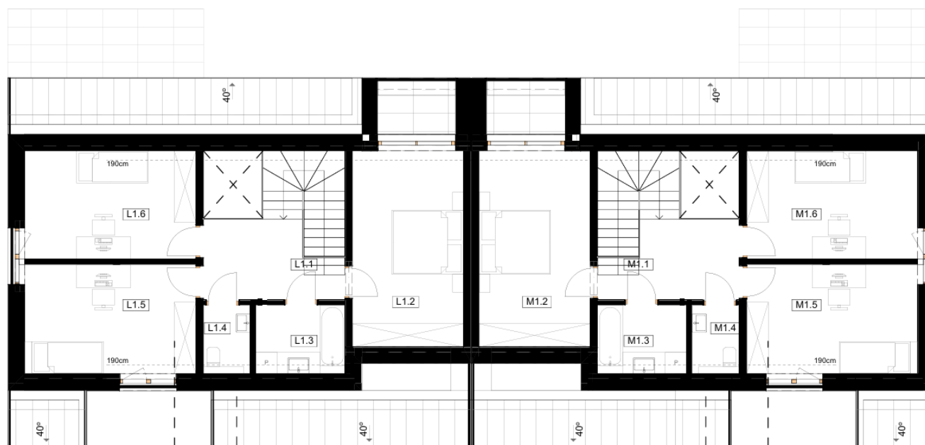
RZUT PODDASZA
