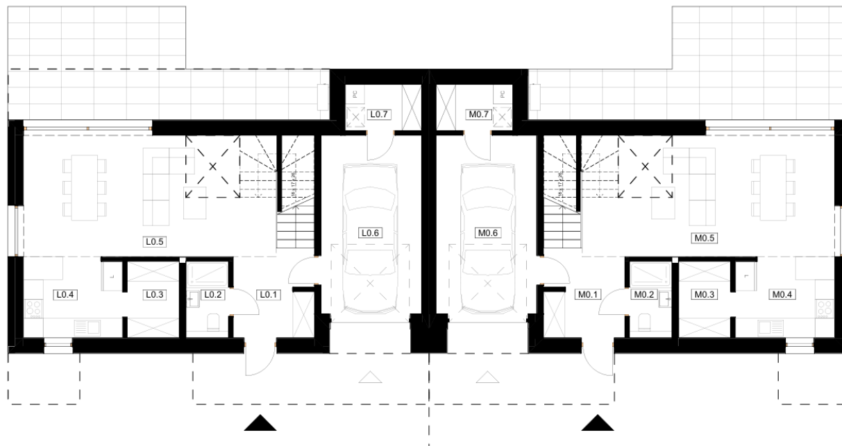
RZUT PARTERU
